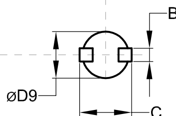
Габаритные и присоединительные размеры, [мм]
