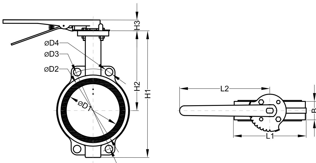
Габаритные и присоединительные размеры, [мм]
